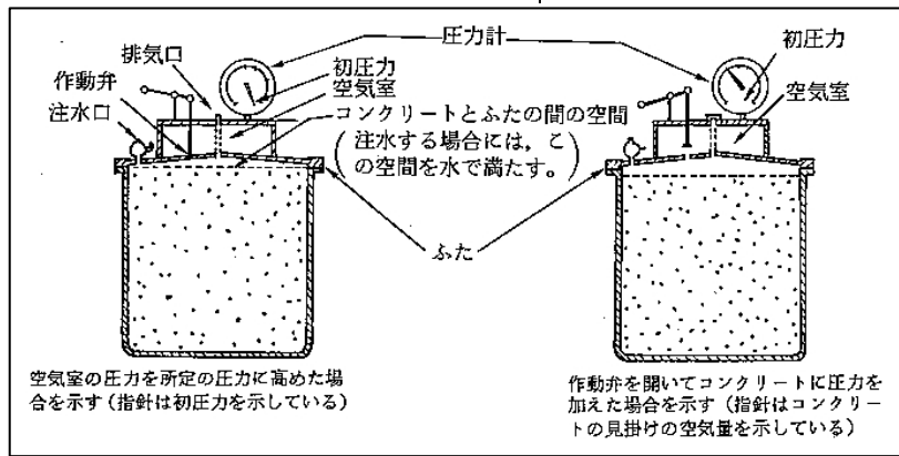
図5-6 空気室圧力方法 (ワシントン型エアーマーター)
